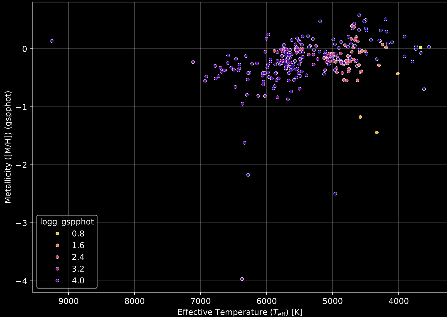
APOGEE DR17 Field: [054-35_MGA] Stellar Population Parameters (n= 270)
